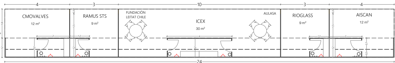
PLANTA
