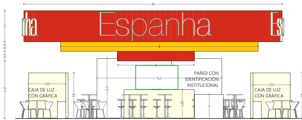
A 01 - ALZADO OESTE - FRONTAL
