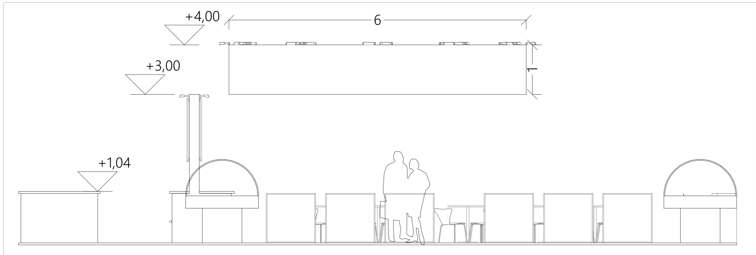
ELEVATION A
