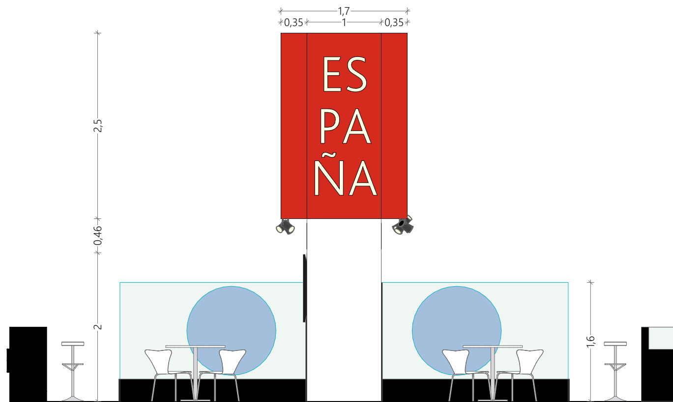
Elevation E3
