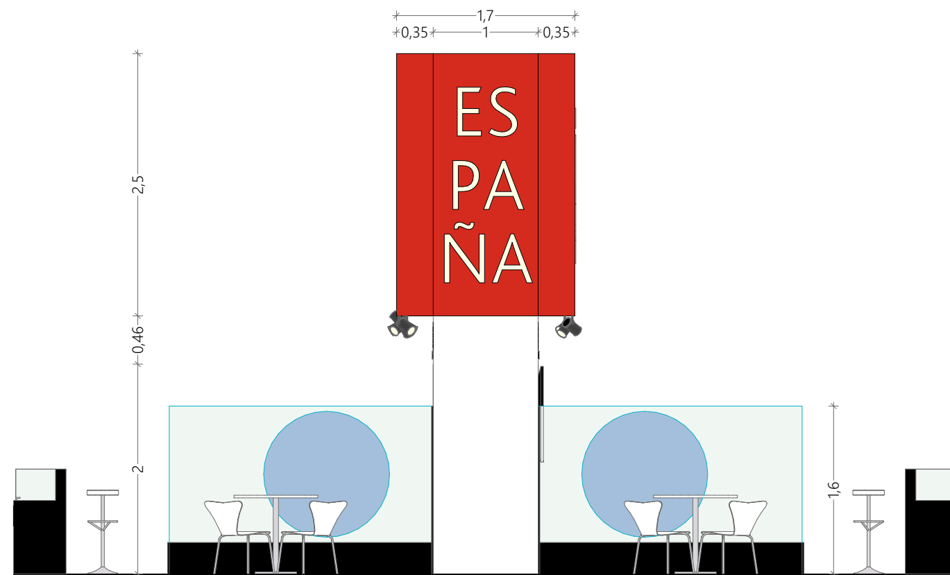
Elevation E4
